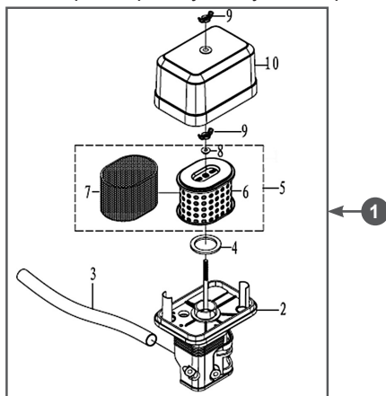
Рис.22 Устройство воздушного фильтра
