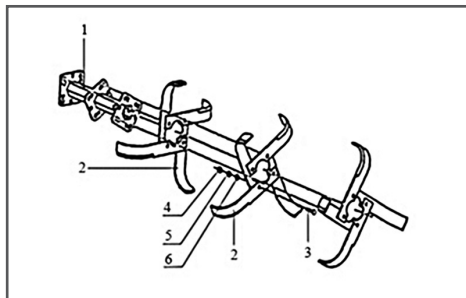
Рис.11 Сборка фрез
