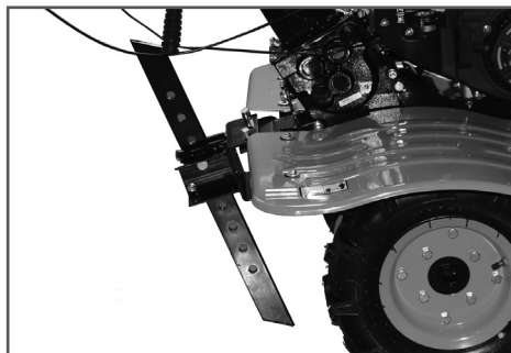
Рис.4 Установка сошника
