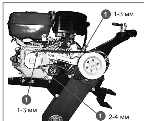
Рис. 10 Регулировка расстояния между ремнем и ограничительными скобами
