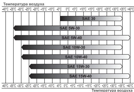
Рис. 13 Определение вязкости масла
