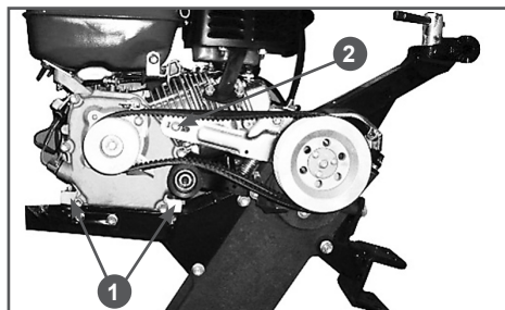
Рис. 9 Регулировка натяжения ремня привода
