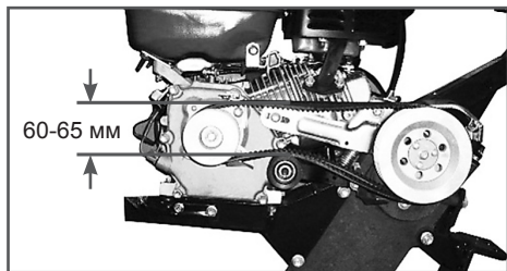
Рис. 8 Параметры натяжения ремня привода
