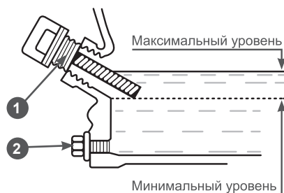
Рис. 14 Проверка уровня масла в картере
